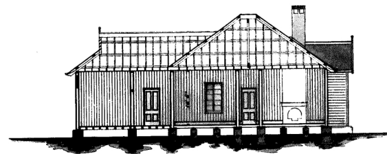
SECTION AB.
